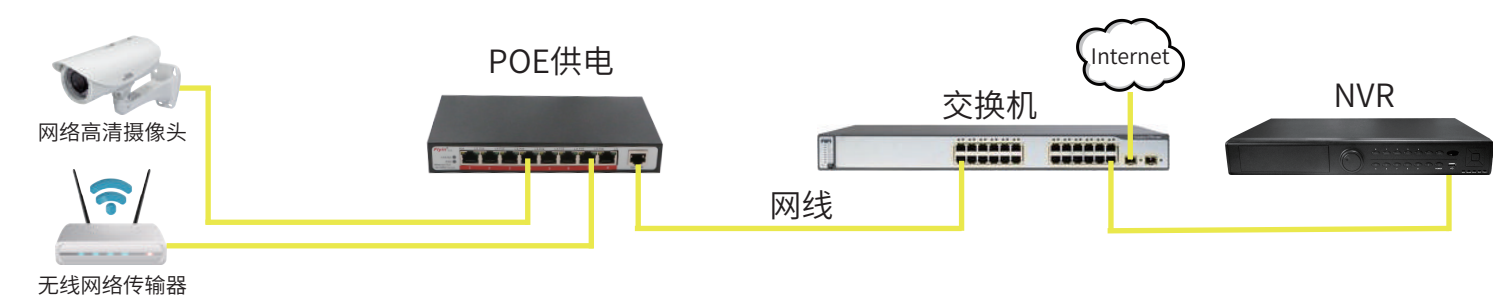
产品连接图
